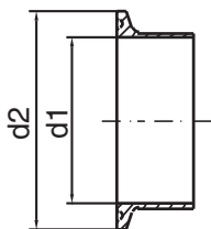
ISO 2852
