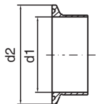
DIN 32676
