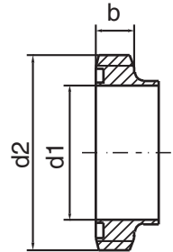
SMS 1145
