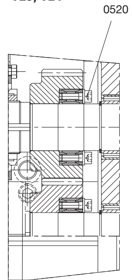
TL3, TL4
