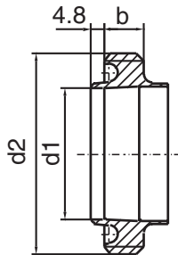
DS 722
