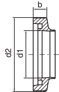
SMS 1145
