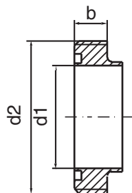
DS 722
